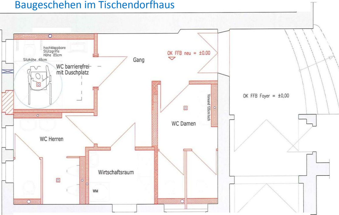
Grundriss des neu entstehenden Sanitärtraktes
